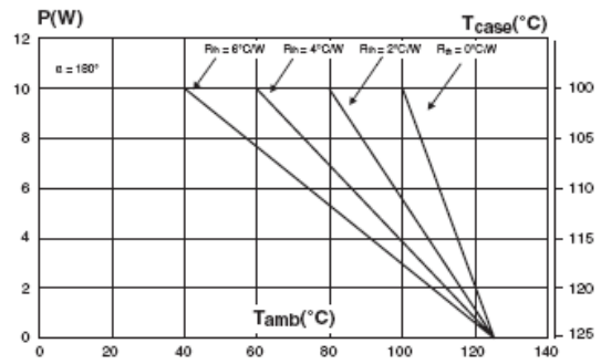
图 2. 最大平均功耗对最大允许温度
