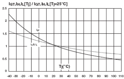
图 5. 触发电流对结温
